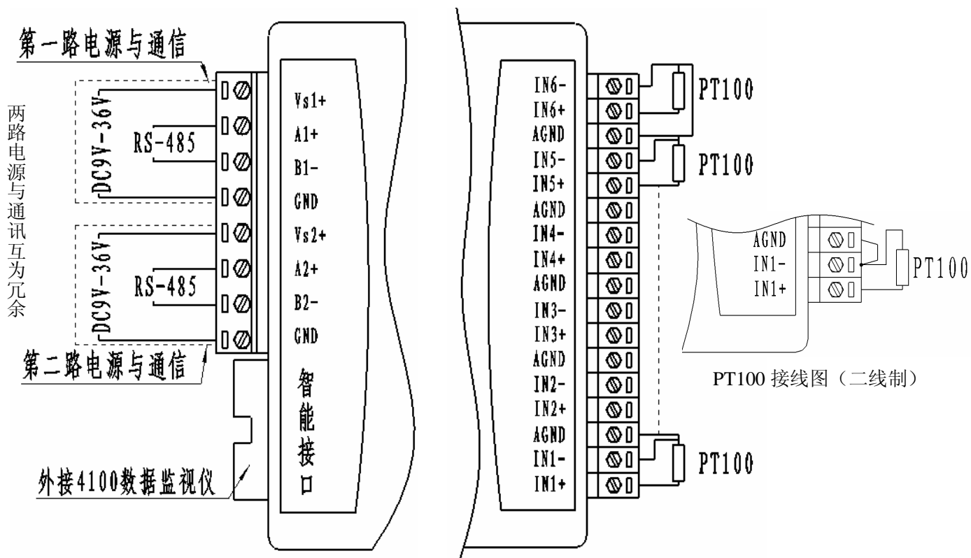
电源、通讯接线图
