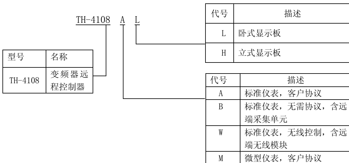
(图 3-1) 变频器远程控制器型号说明
